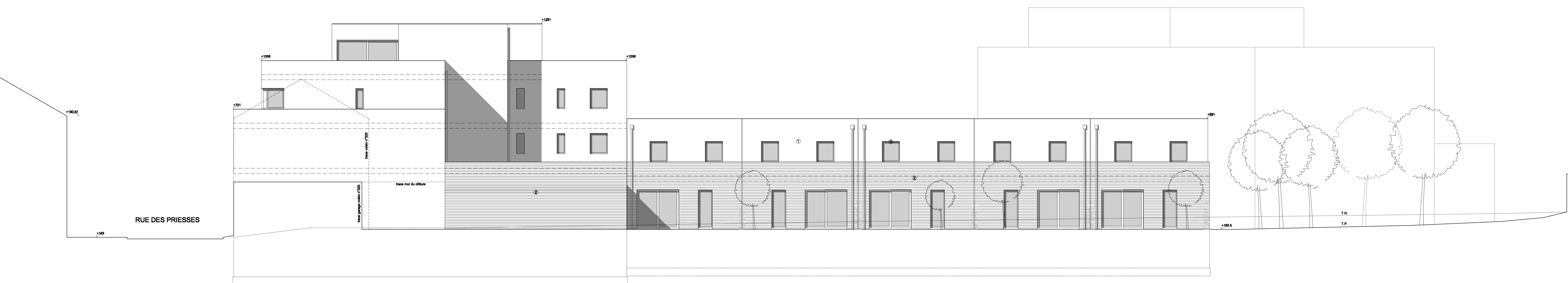
ELEVATION SUD-EST IMMEUBLE B et C échelle 1/100
