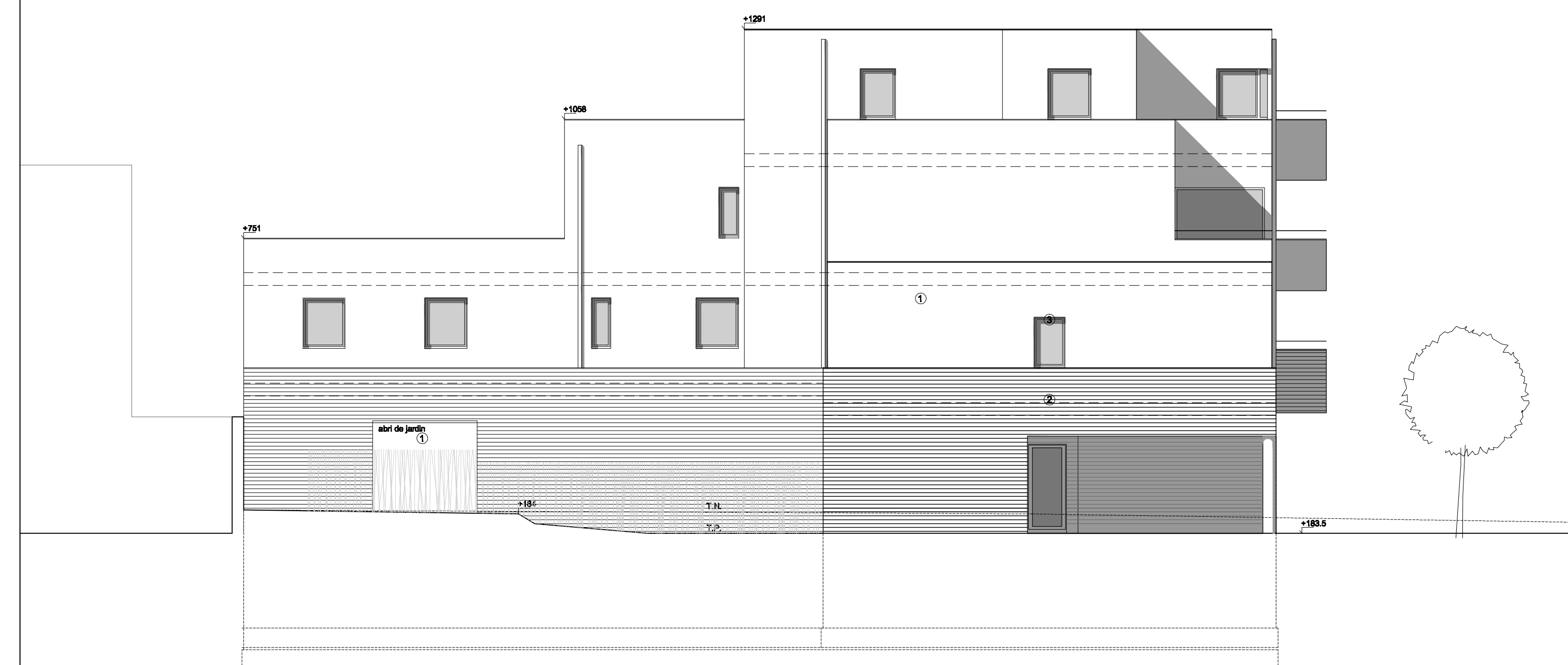
ELEVATION NORD-EST IMMEUBLE B et C échelle 1/100
