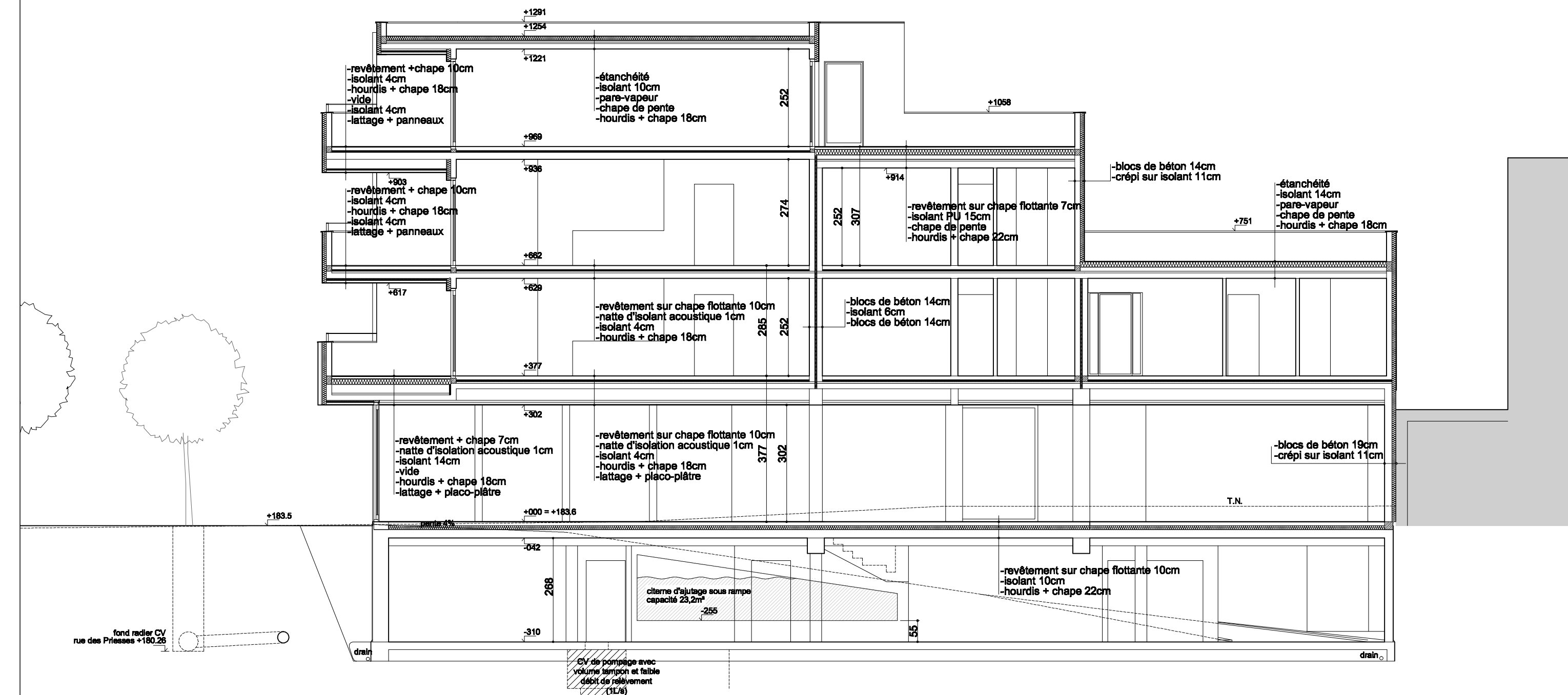
COUPE DD IMMEUBLE B et C échelle 1/100
