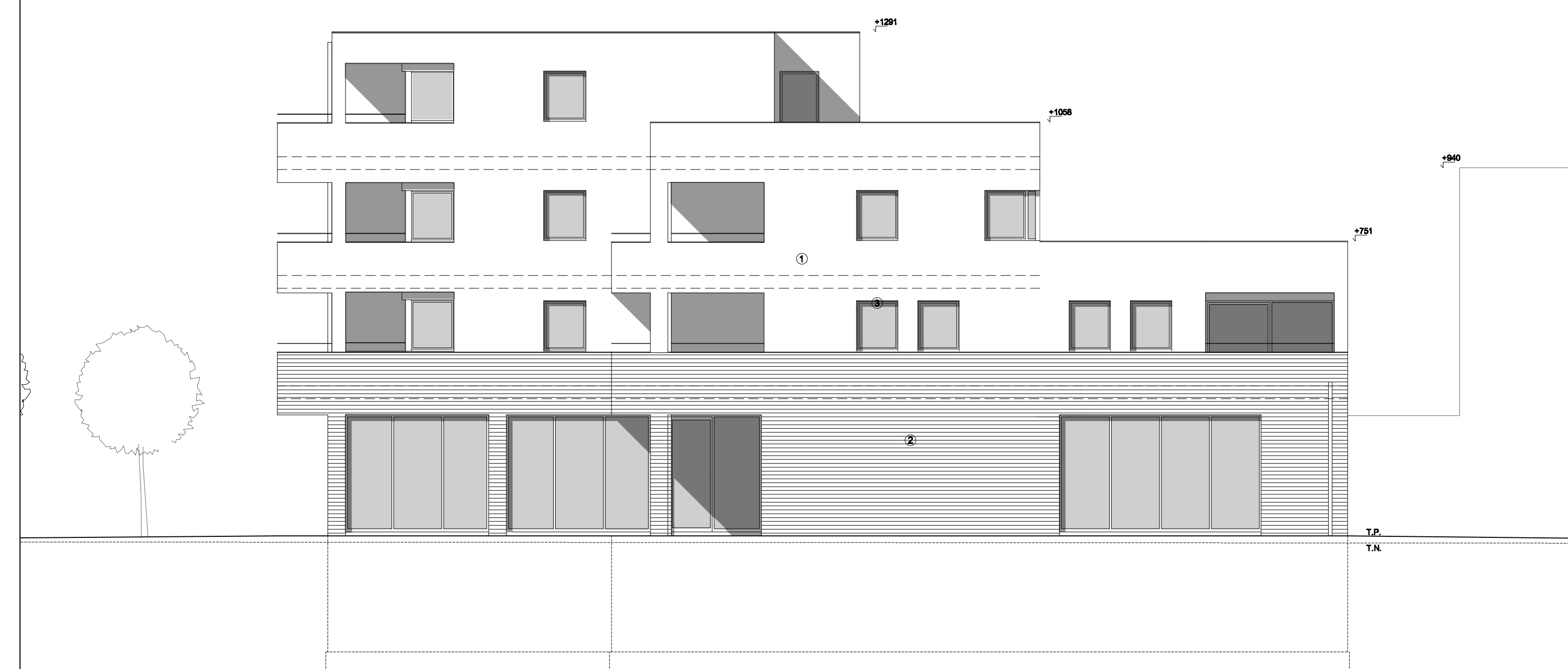
ELEVATION SUD-OUEST IMMEUBLE B et C échelle 1/100
